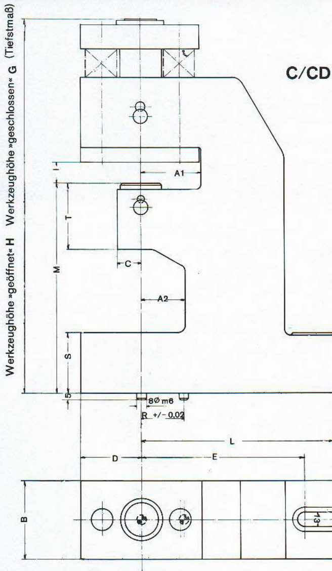
Maßtabelle C/CD
